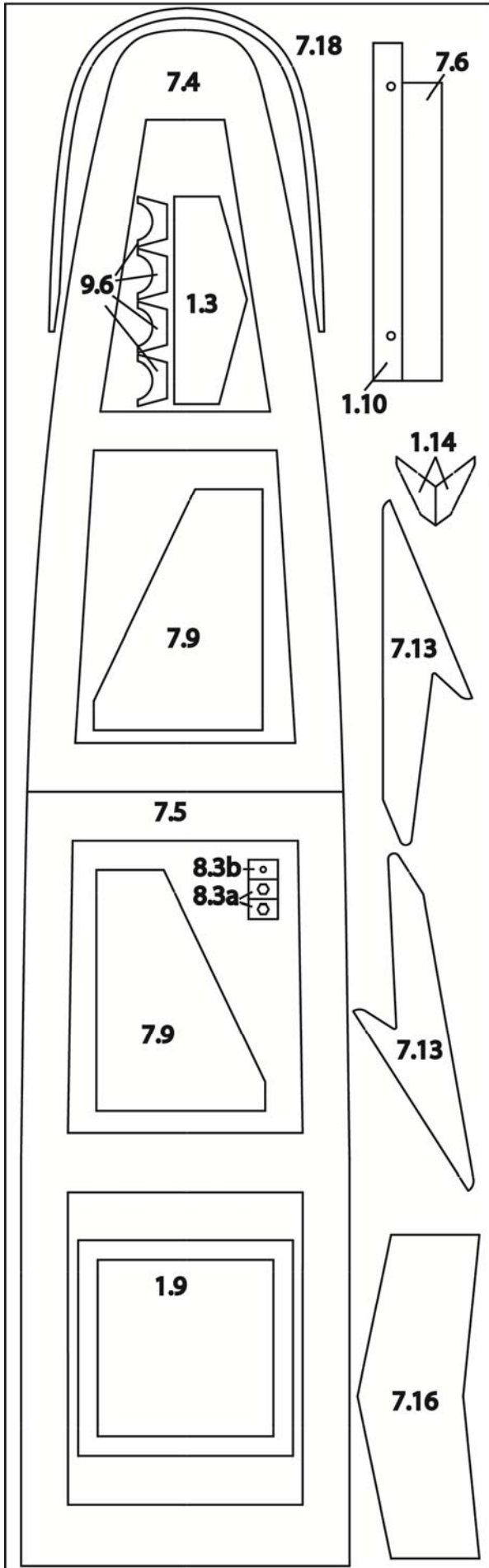
Laserplatte 4
